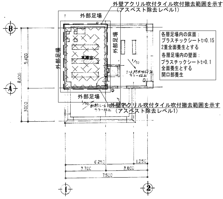
搭屋 1階平面図 1:100
