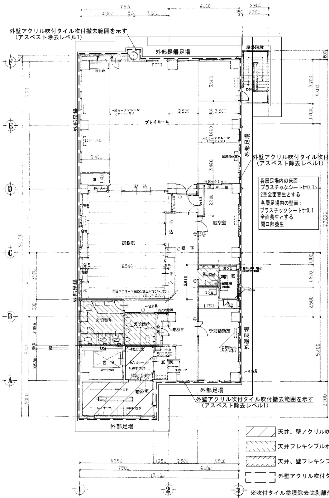
5階平面図 1:100
