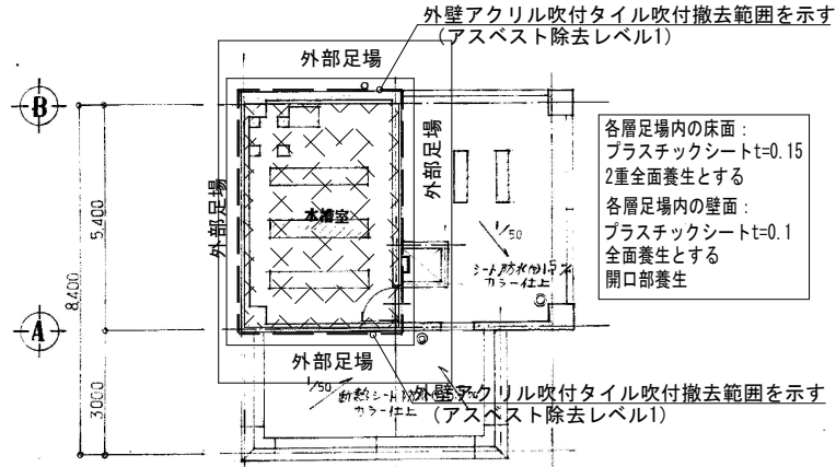
搭屋 2階平面図 1:100
