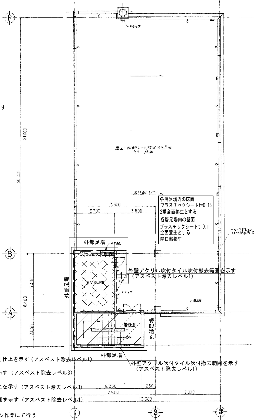
5階天井、壁吹付タイル
